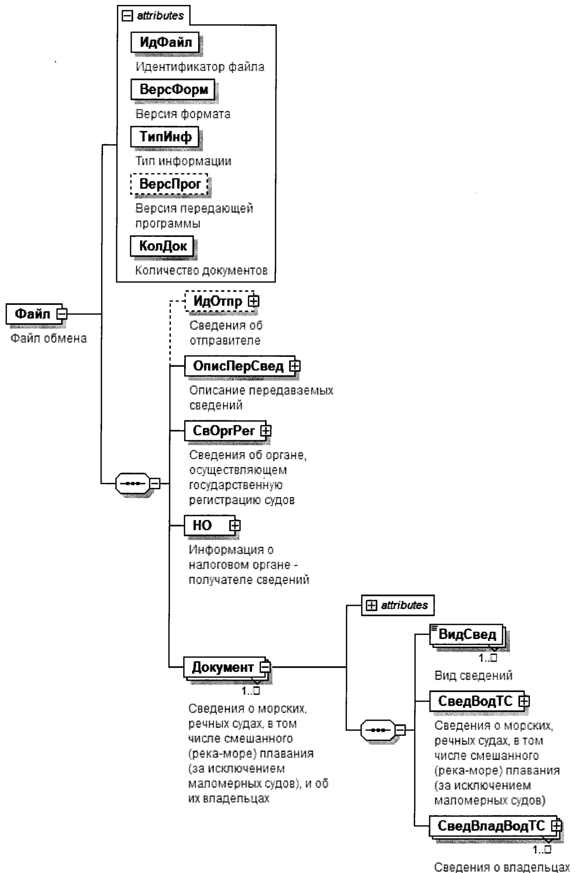
Рис.1. Диаграмма структуры файла обмена
